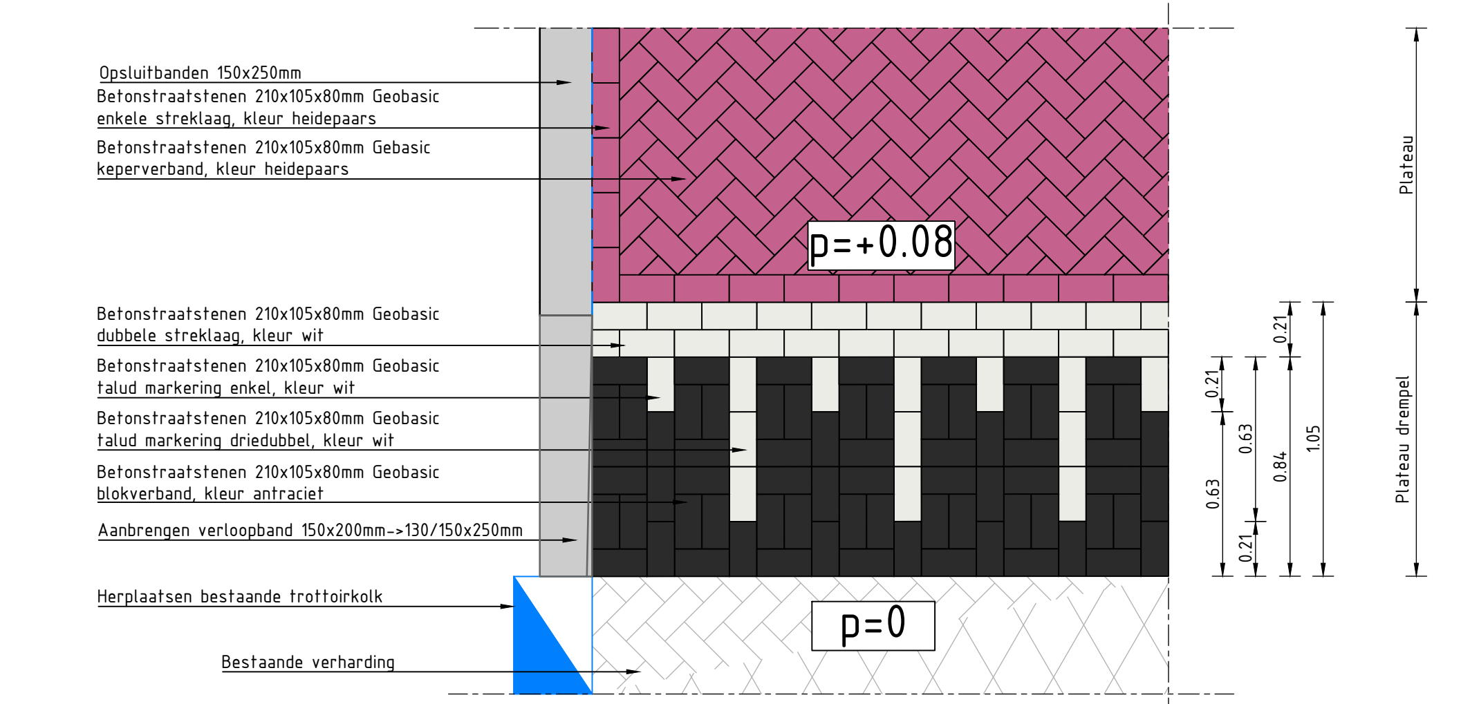
DETAIL PLATEAU DREMPEL
