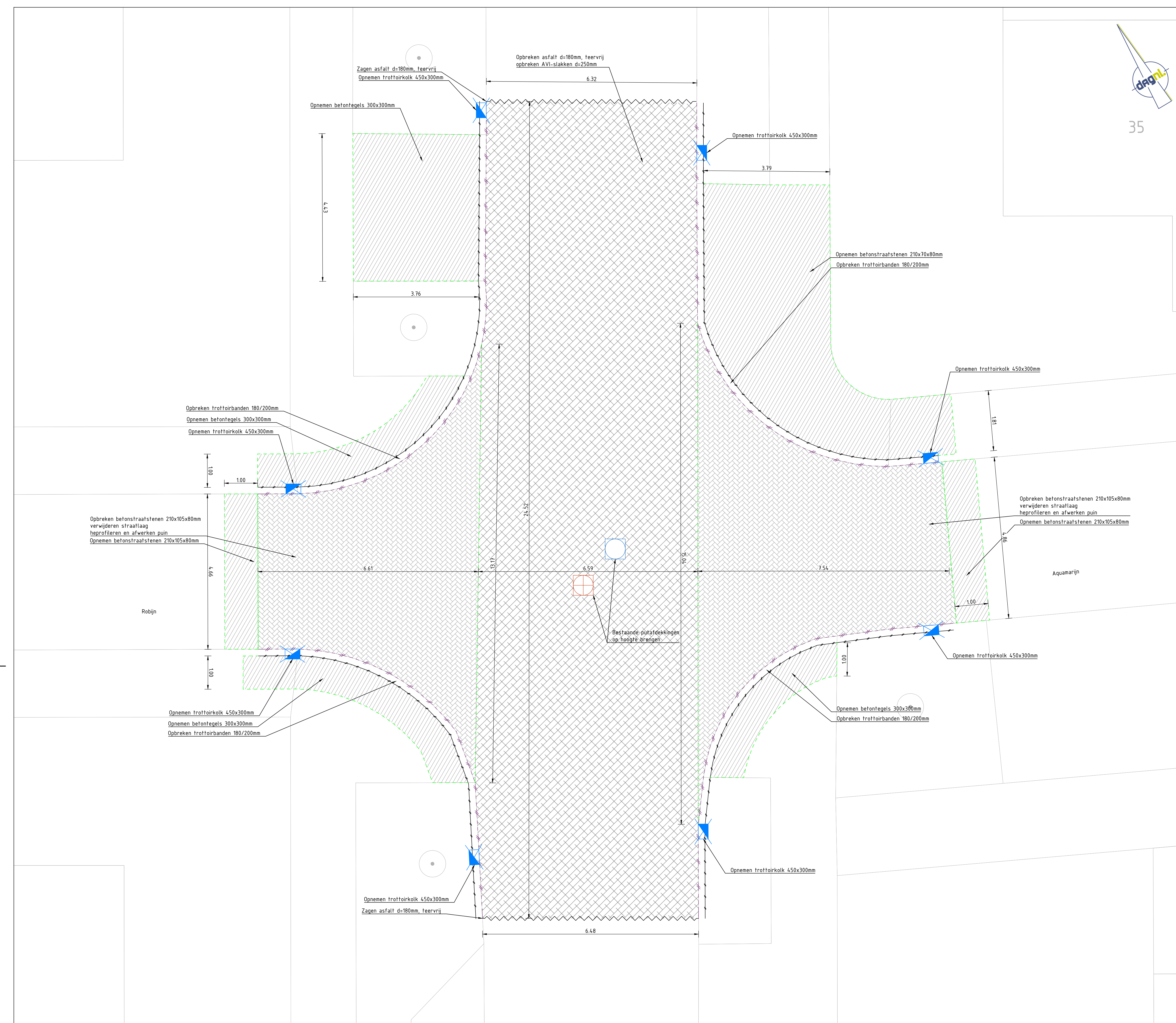
LOCATIE 2: SITUATIE OPBREKEN PLATEAU
