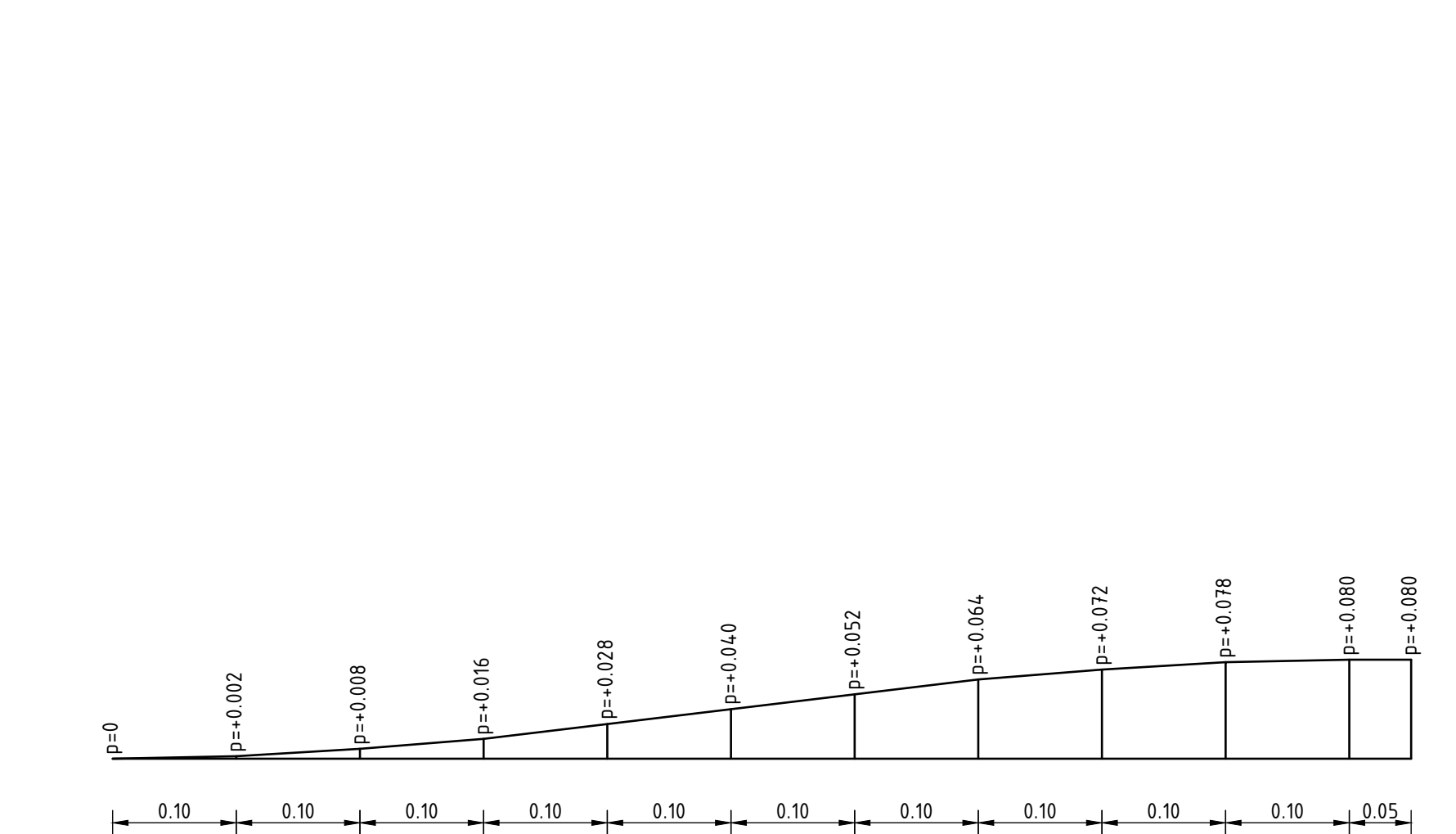
DETAIL HOOGTEVERLOOP PLATEAU DREMPEL
